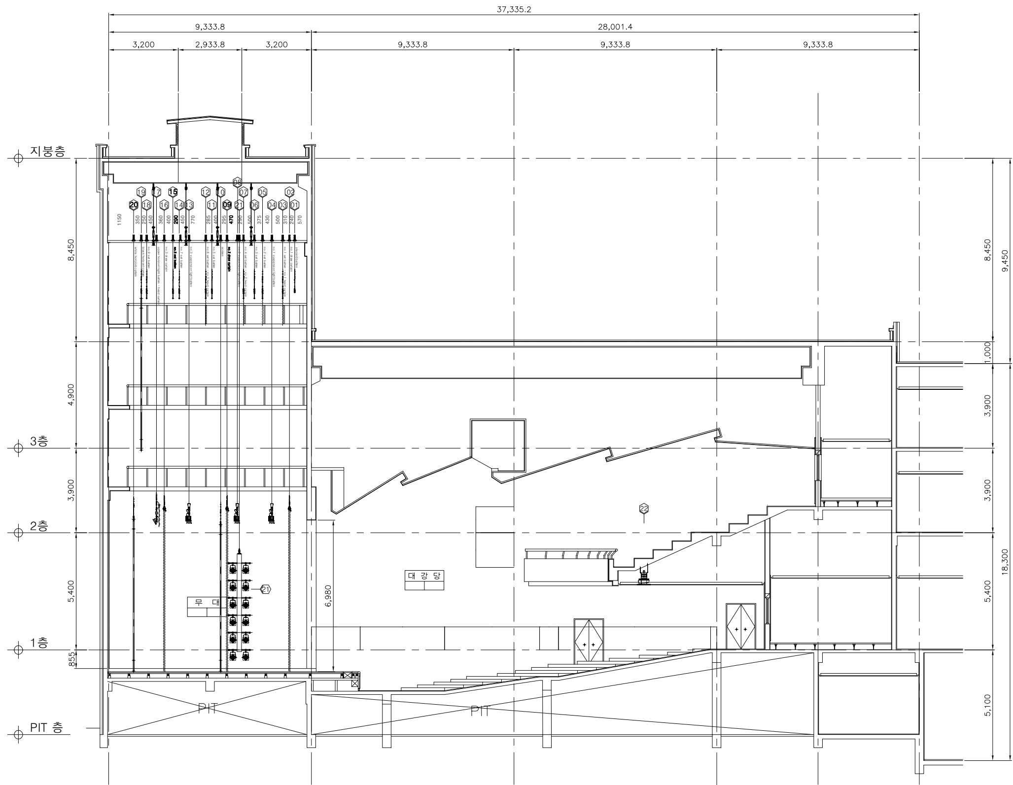
1 대공연장 무대기계 단면도 축척 : 1/160
